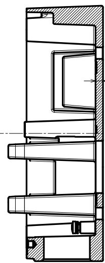
SecB-B
