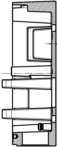
SecB-B
