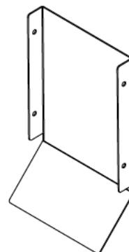
ボックスカバー×1
